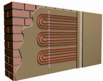
Lehmputz in Verbindung mit WEM-Wandheizung
